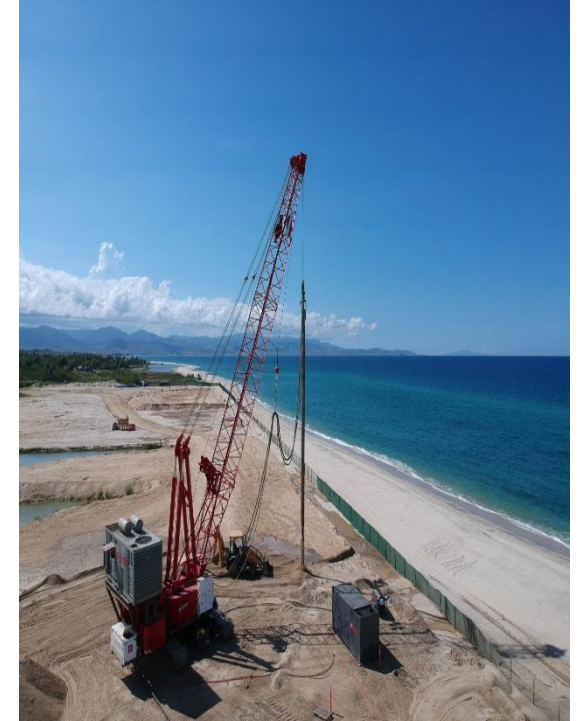
Vibro Compactación
