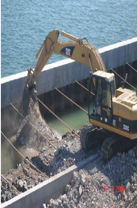
Trabajos de reclamación de terreno al mar.
