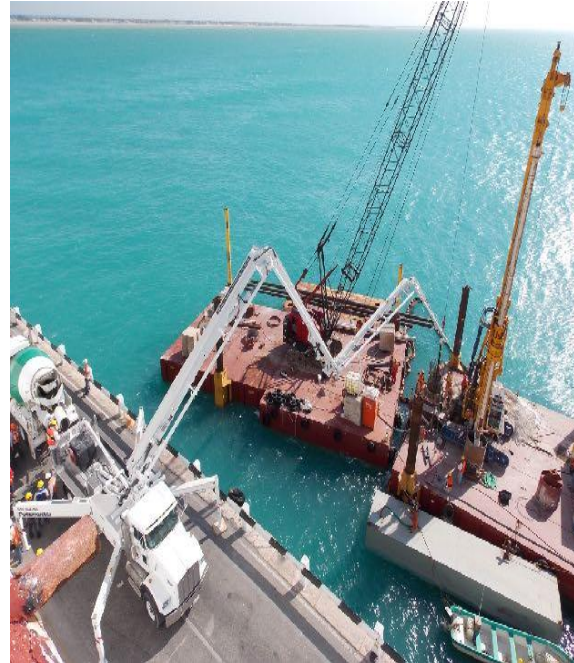
Cimentación Marina sobre barcas e hincado de pilotes.
