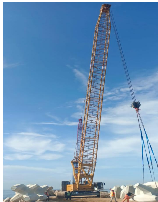
Colocación de Core-Lock
